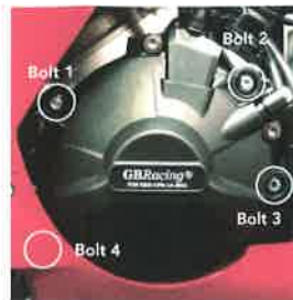
Bolt 4 M6X35HHF - 10Nm
