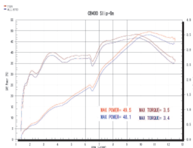
Slip-On チタン φ115-350
